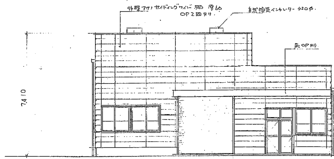
北立面图
