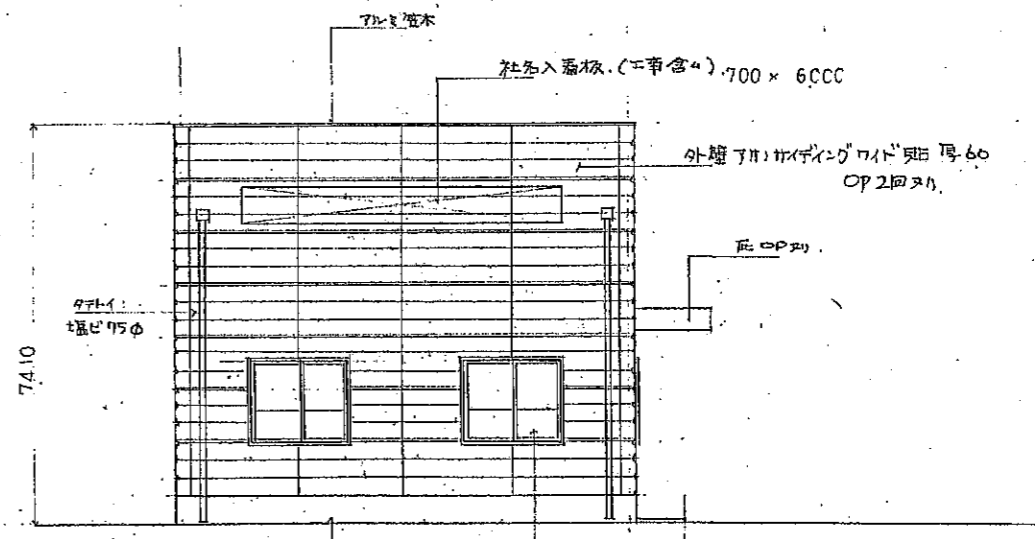
東立面图
