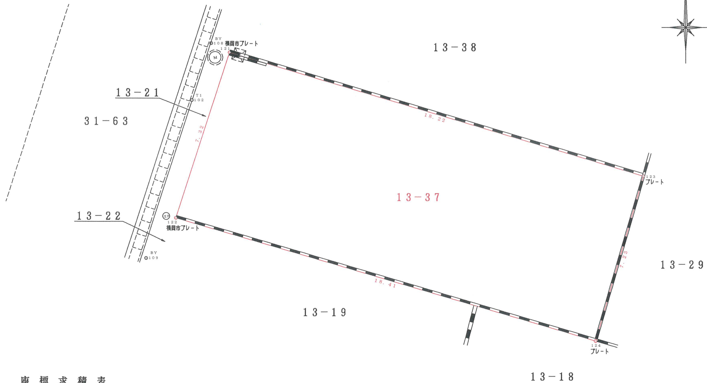
地 番 NO 標 識 X Y 辺 長 測 線 13 121 ( ) 70796.635 -49992.061 -37 122 ( ) 70789.663 -49994.310 7.32 121- 122 124 ( ) 70784.513 -49976.630 18.41 122- 124 123 ( ) 70791.457 -49974.590 7.23 124- 123 121 ( ) 70796.635 -49992.061 18.22 123- 121 倍面積 266.729054 m 2 面 積 133.3645270 m 2 地 積 133.36 m 2 坪 数 40.3427
