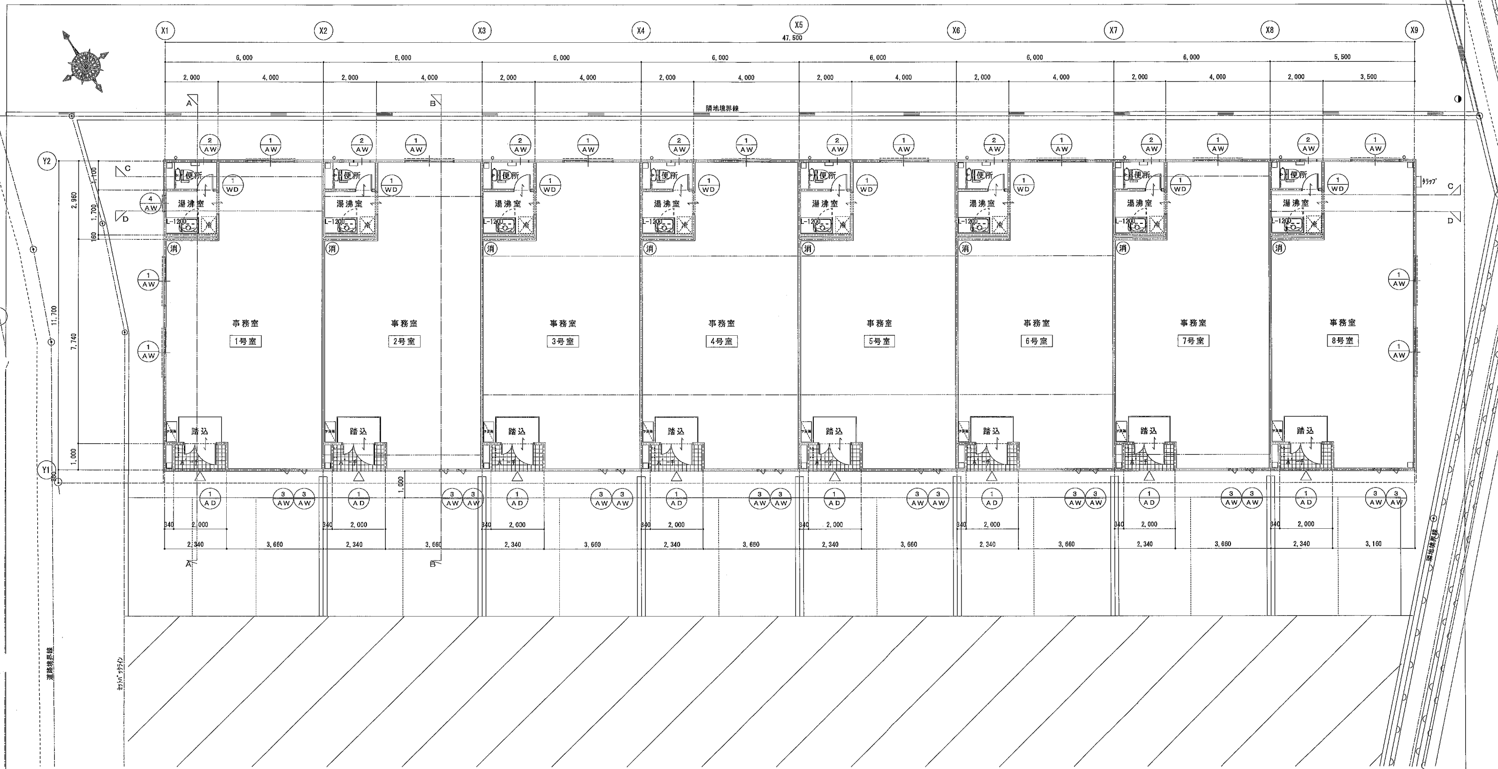
平面図 S = 1 : 100
