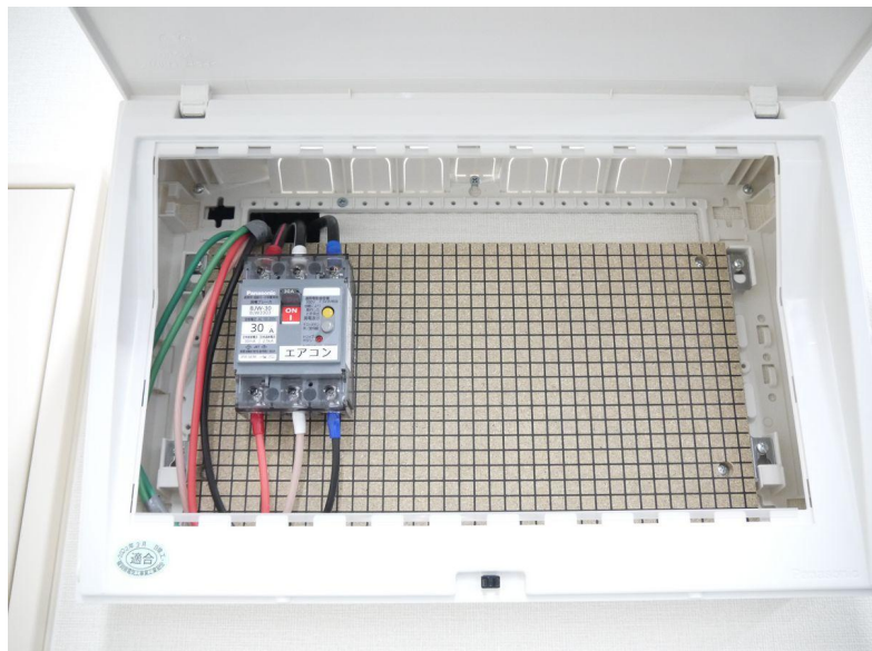
事務室 動力分電盤
